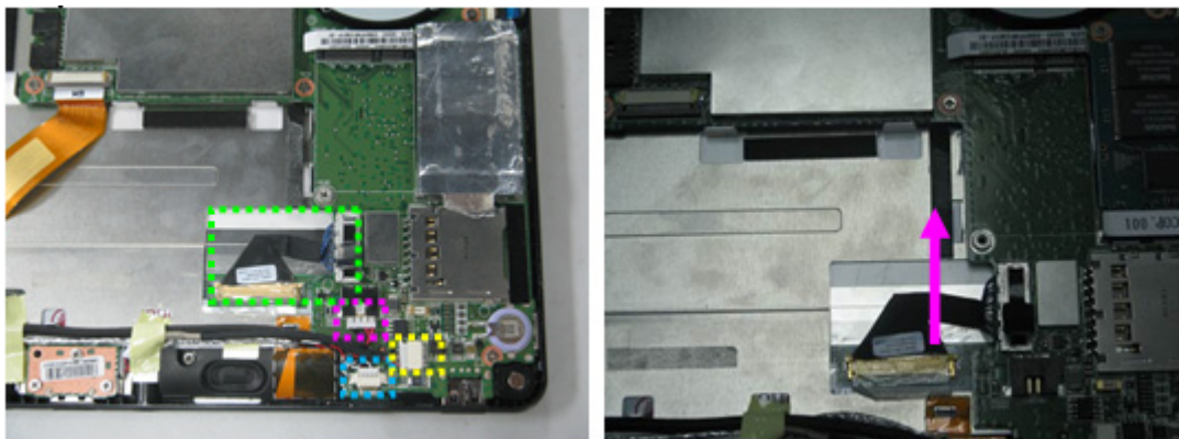
Figure 3-5. Mini Card
