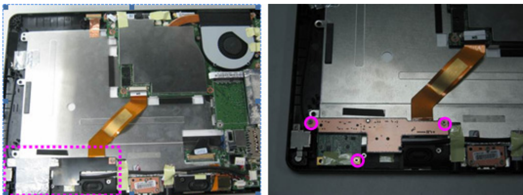
Figure 3-6. Mini Card
